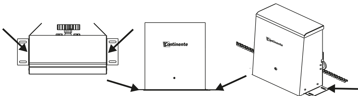
Figura 01: Fixar as base do Kit ao corpo do Movimentador Deslizante
